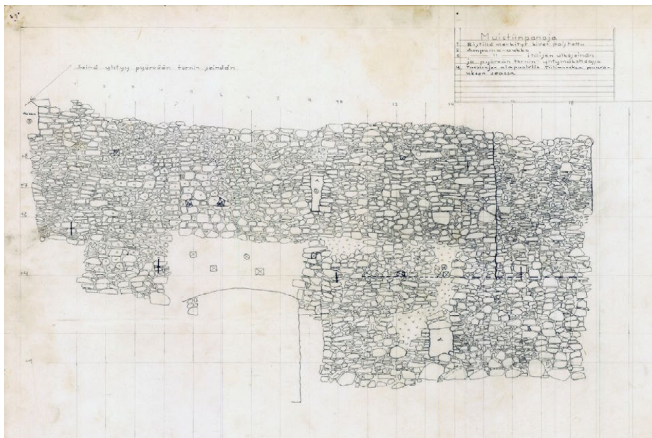
Kuva 15. Ote vuoden 1961 mittauspiirustuksesta, jossa on esitetty vuoden 1962 restauroinnissa havaittu vaakatasoinen muurisauma. Piirros: Veijo Laine 1961. Museoviraston arkisto, Rakennetun kulttuuriympäristön piirustukset KYP835020051. Kuvankäsittely: Tarja Knuutinen.
