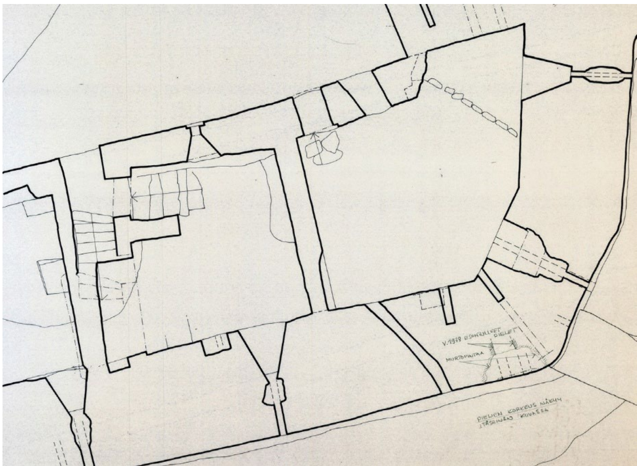
Kuva 10. Mittauspiirros vuonna 1978 itäisen kehämuurin pohjoisosan romahduksesta ja sen alta paljastuneista "pielistä". Piirros: Tekijä tuntematon 1978. Museoviraston arkisto, Rakennetun ympäristön piirustukset, KYP2000000014. Kuvankäsittely: Tarja Knuutinen.
