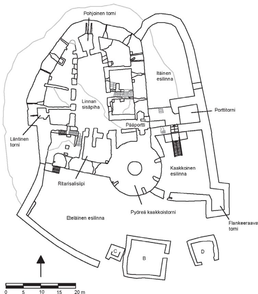
Kuva 1. Raaseporin linnan pohjakartta ja tekstissä mainitut linnan pääosat. Pohjakartta: Metsähallitus 2024.
