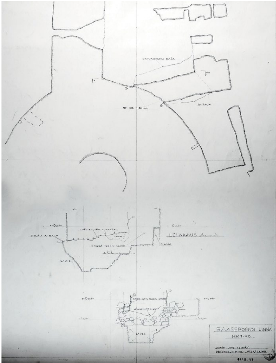
Kuva 16. Mittauspiirros Ritarisalisiiven itäseinän kaivauksesta ennen perustusten vahvistamista. Piirroksessa esitetty Ritarisalisiiven itäseinän ja pyöreän tornin muurin välinen suhde. Piirros: Veijo Laine 1962. Museoviraston arkisto, Rakennetun ympäristön piirustukset KYP835020047. Kuvankäsittely: Tarja Knuutinen.
